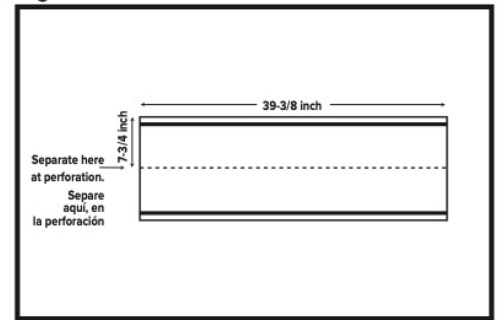
Fig. 1 Shingle Starter Teja de la hilera inicial
