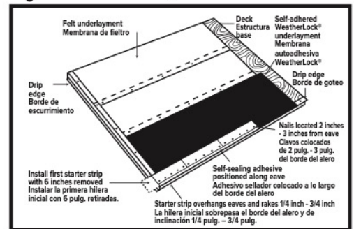
Fig. 2 Shingle Starter Application Instalación de tejas de la hilera inicial
